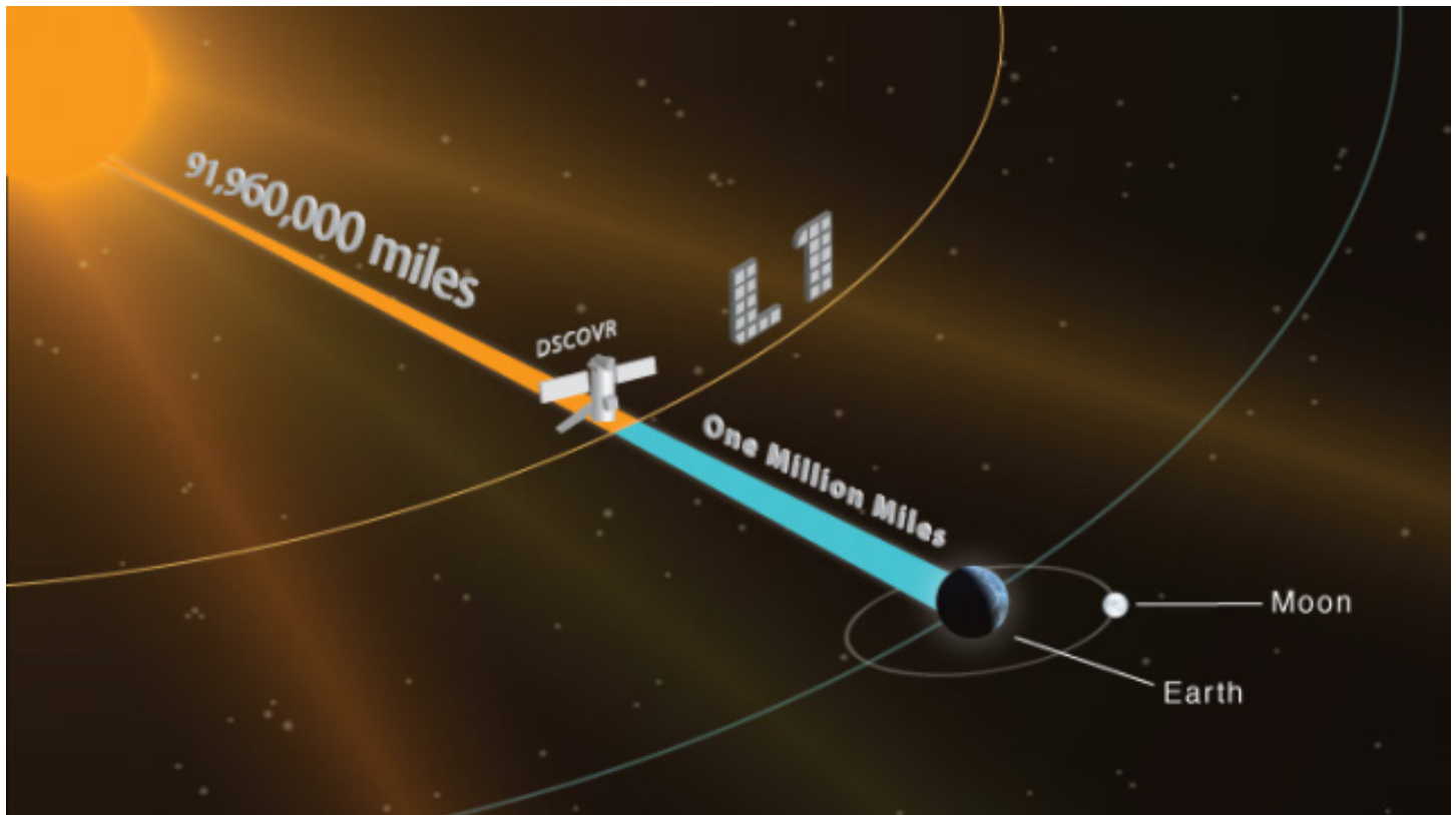
DSCOVR
