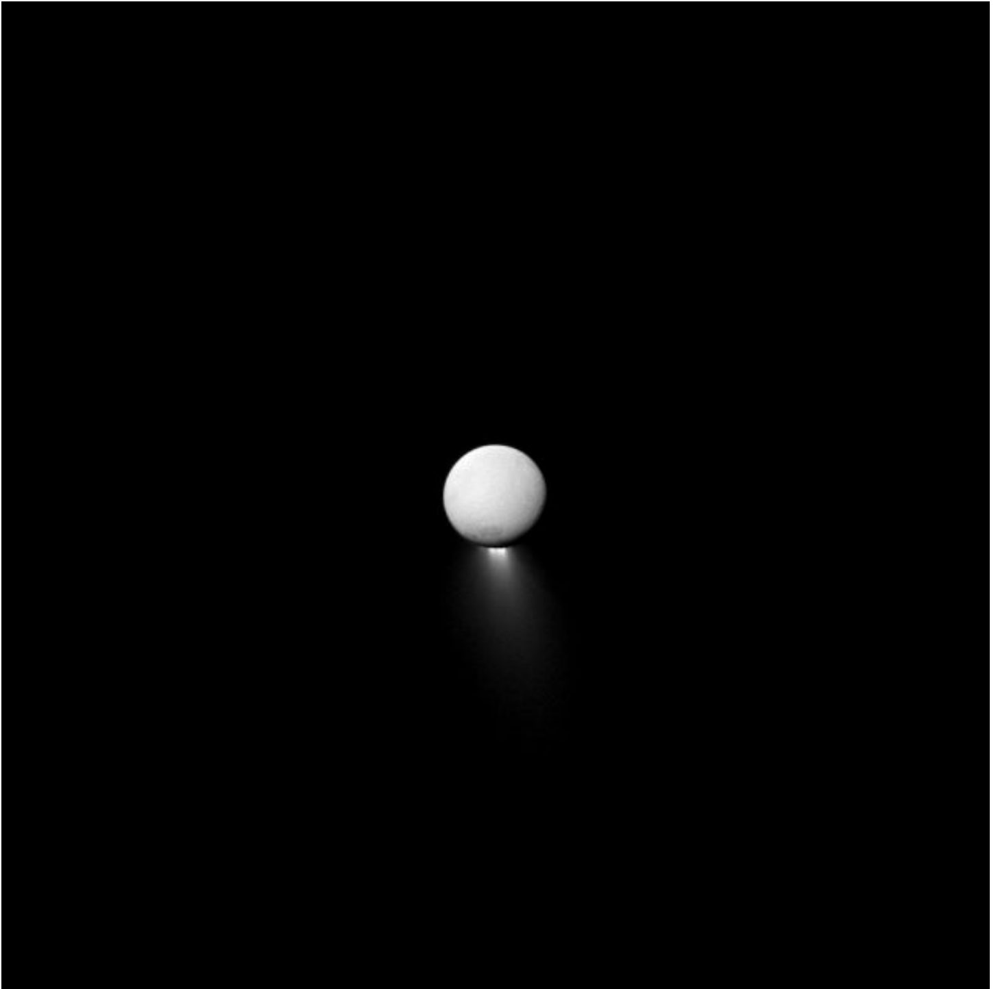
Enceladus
